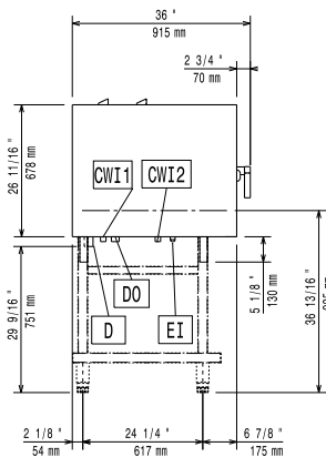
Zij aanzicht
